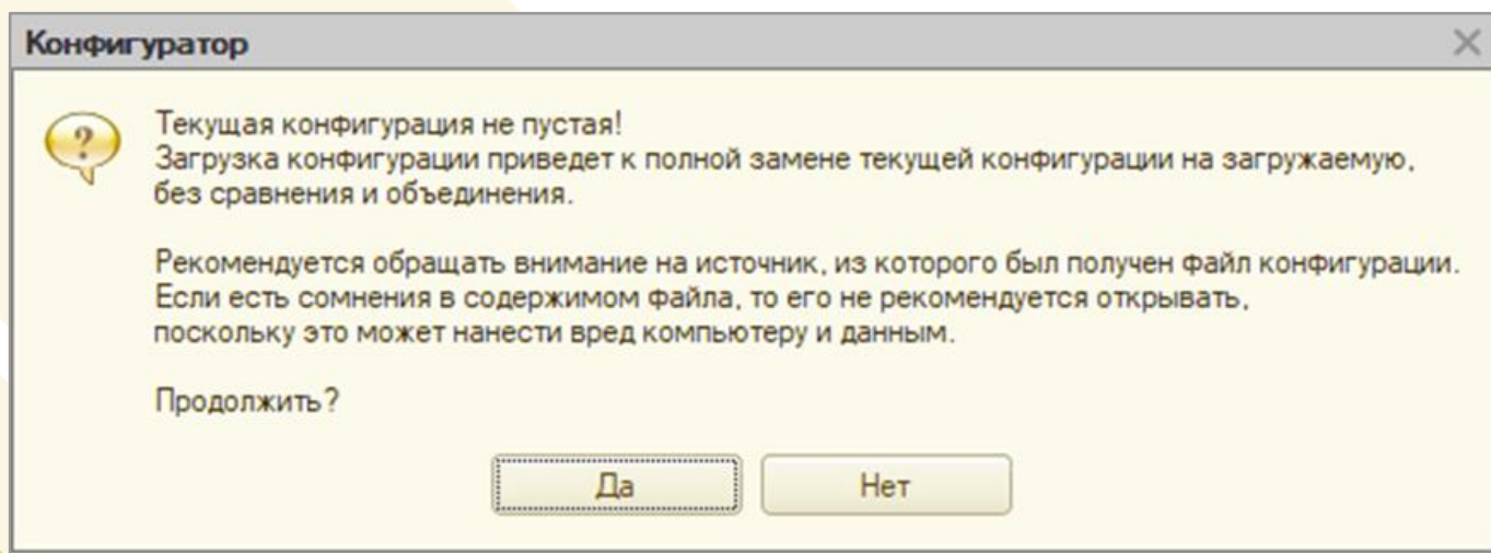
Рисунок 15 - Предупреждение
