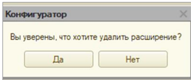
Рисунок 31 - Предупреждения удаления
