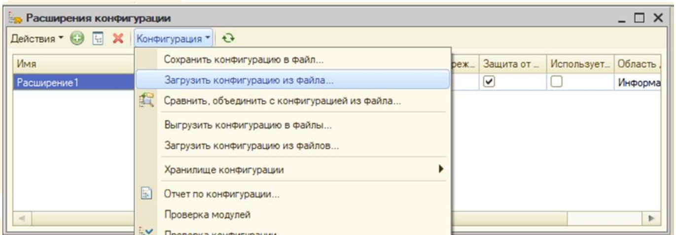
Рисунок 4 - Загрузка расширения
