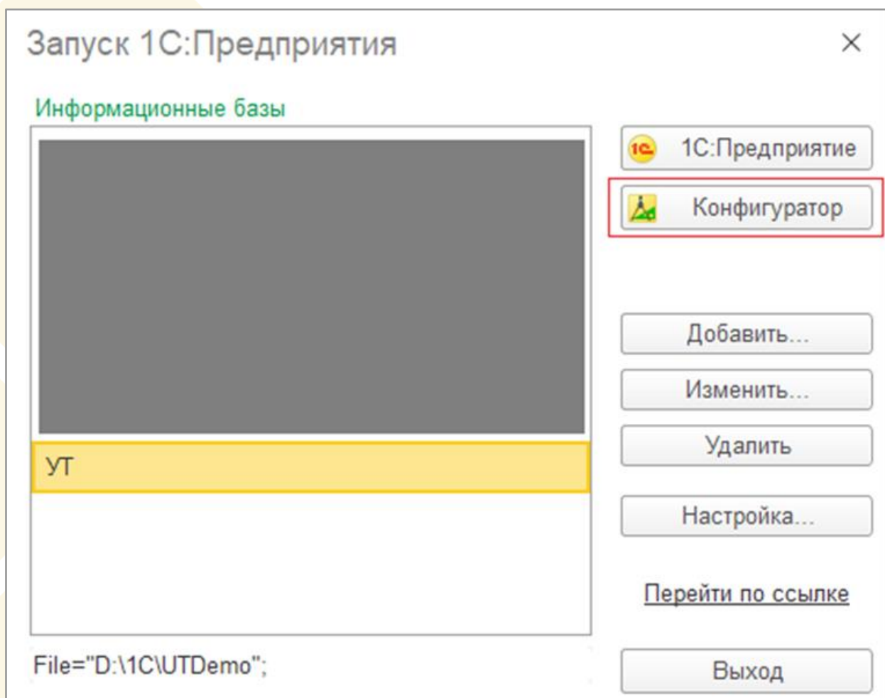
Рисунок 27 - Запуск платформы
