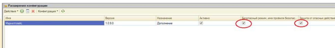
Рисунок 17 - Режимы расширения
