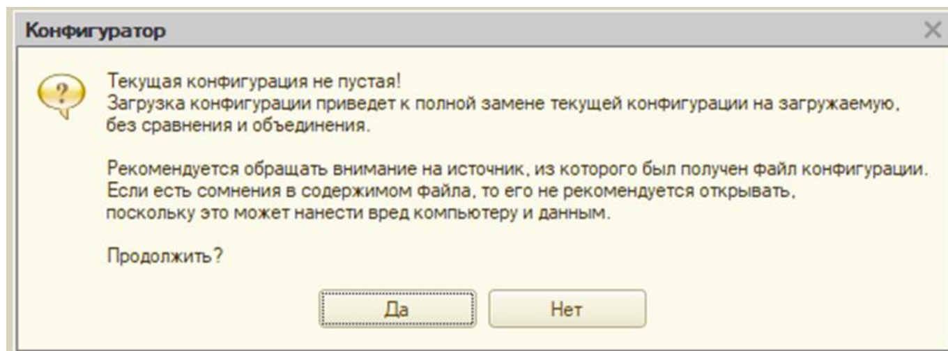
Рисунок 5 - Предупреждение загрузки
