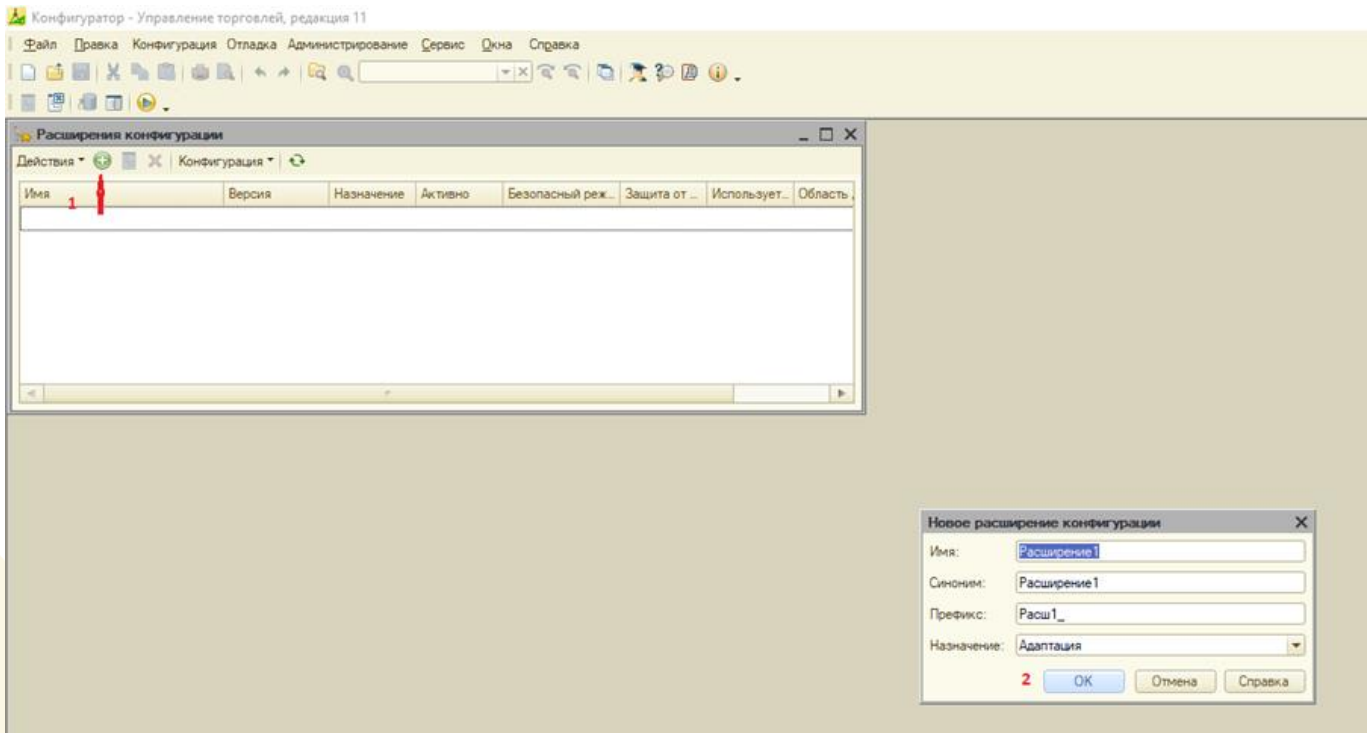
Рисунок 3 - Добавление расширения
