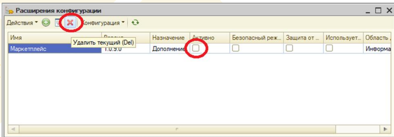
Рисунок 30 - Режимы расширения
